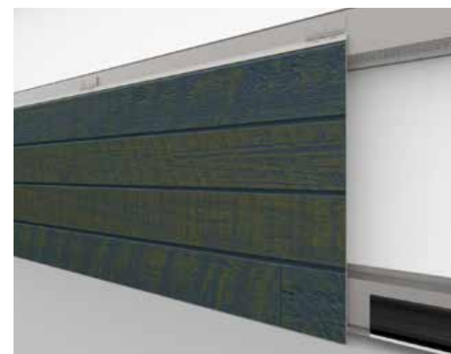
EX series 16 x 455 x 3 030 mm med MolaVent ventilerad, vågrät underkonstruktion. Monteras på cc 455 mm.
