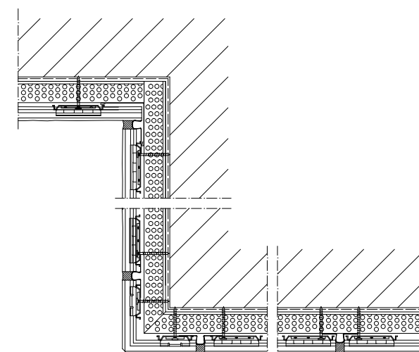
Ritning ovan visar montage med EX-fogmassa och prefabricerade EX-Hörn i matchande utförande och format.
