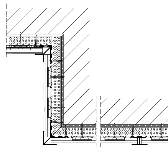
Ritning ovan visar montage med extruderade aluminium hörn- och H-profiler i matchande kulör.
